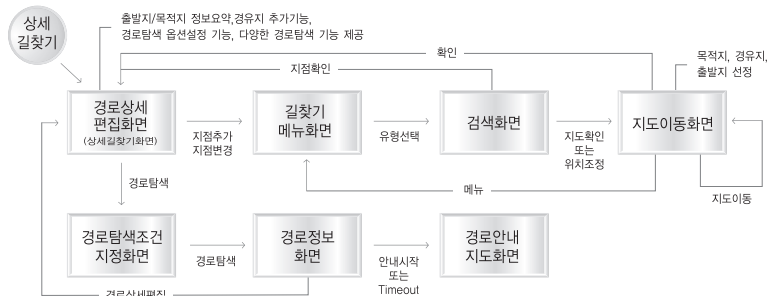
〈 상세길찾기 흐름 요약 (경로상세편집 화면을 통한 경로탐색 흐름 요약) 〉
